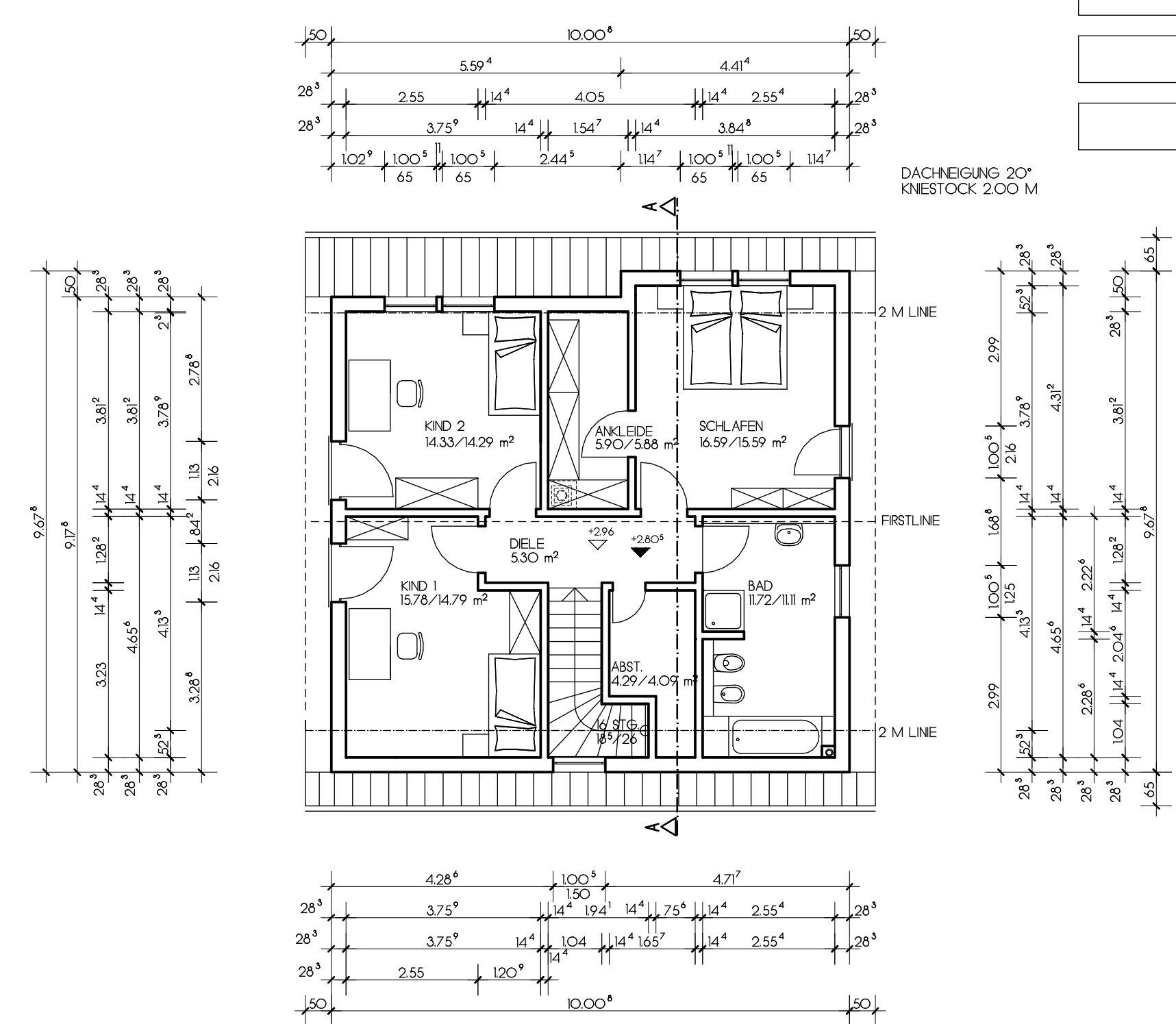
DACHGESCHOSS
